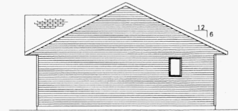
END ELEVATION
